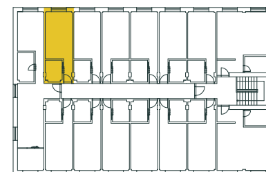
PÔDORYS 2.NP
