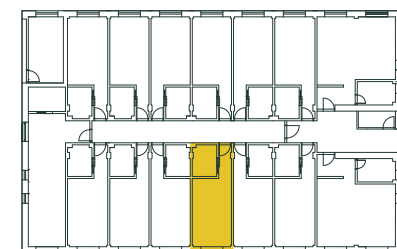
PÔDORYS 1.NP
