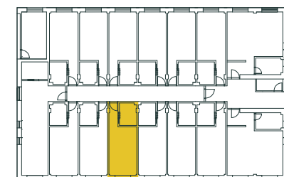
PÔDORYS 1.NP
